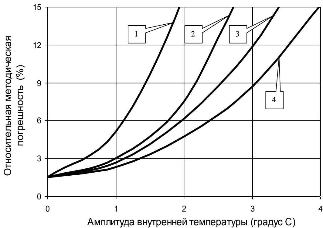
Рис.2. Графики к определению методической погрешности при измерении теплового потока на внутренней поверхности.
