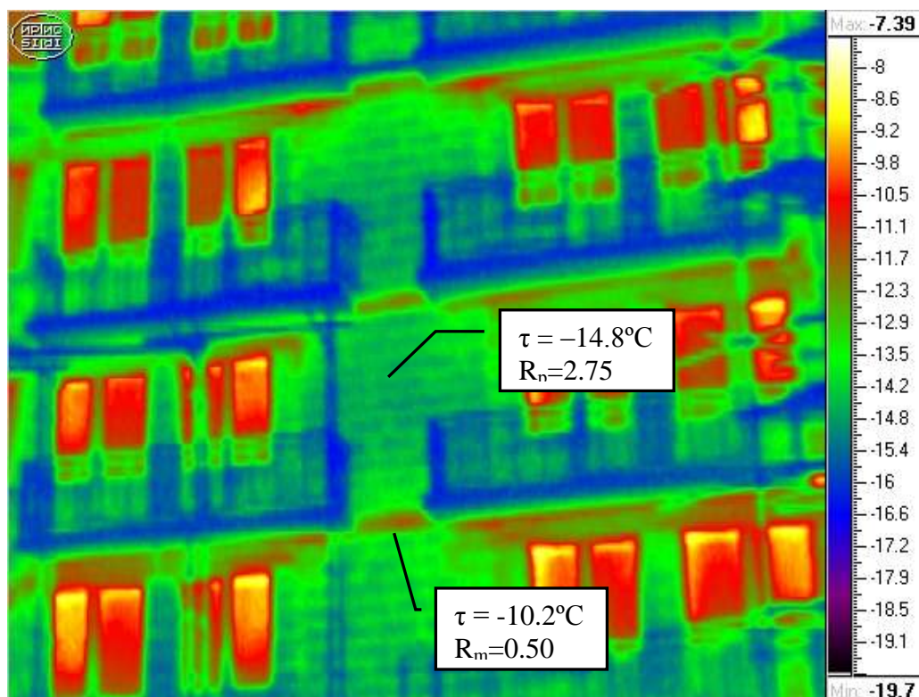
Рис.4. Температура наружной поверхности исследуемых участков определяется по полученным термограммам.
