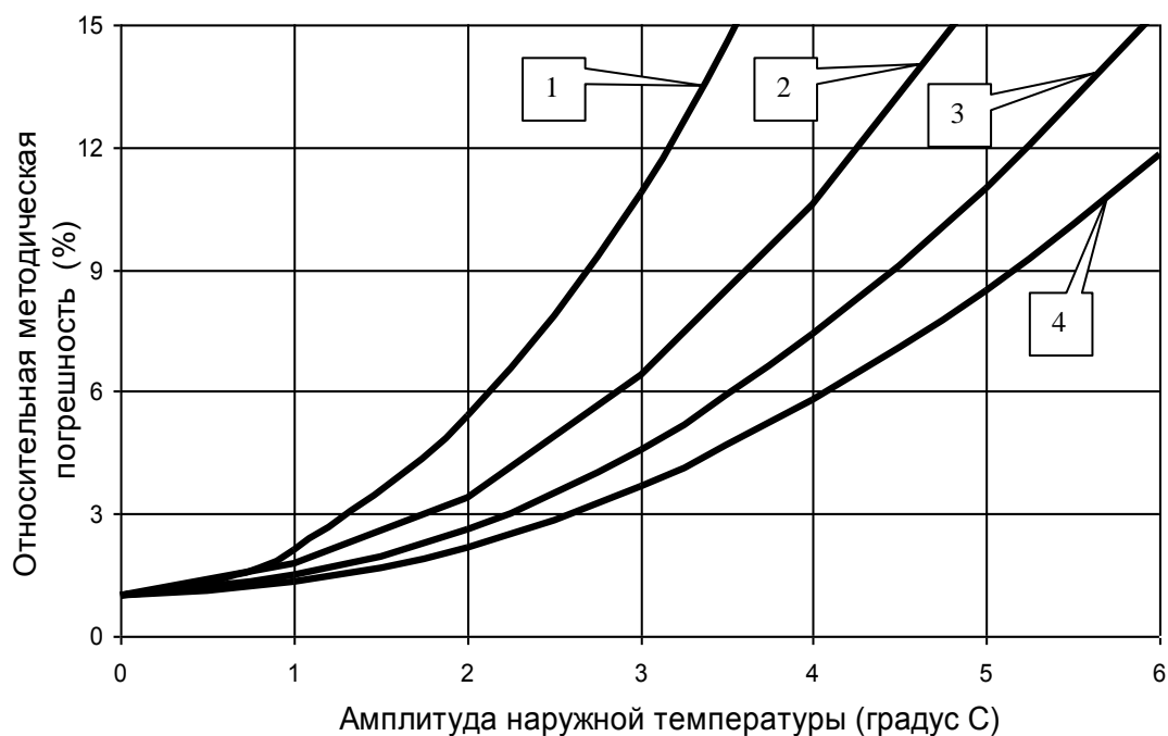
Рис.1. Графики к определению методической погрешности при измерении теплового потока на наружной поверхности.
