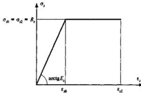
Рисунок 5.2 - Диаграмма состояния растянутой арматуры
