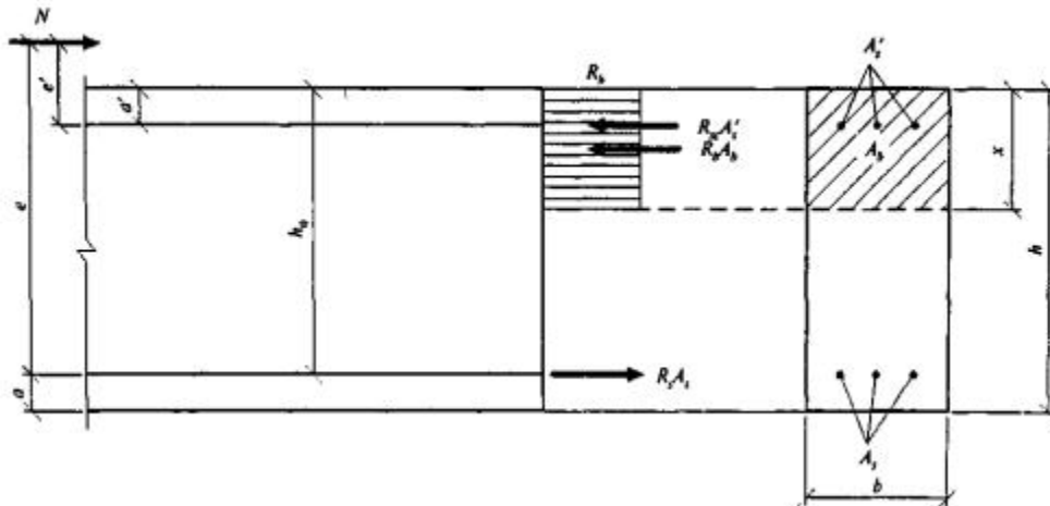
Рисунок 6.5 - Схема усилия и эпюра напряжений в сечении, нормальном к продольной оси внецентренно сжатого железобетонного элемента, при расчете его по прочности
