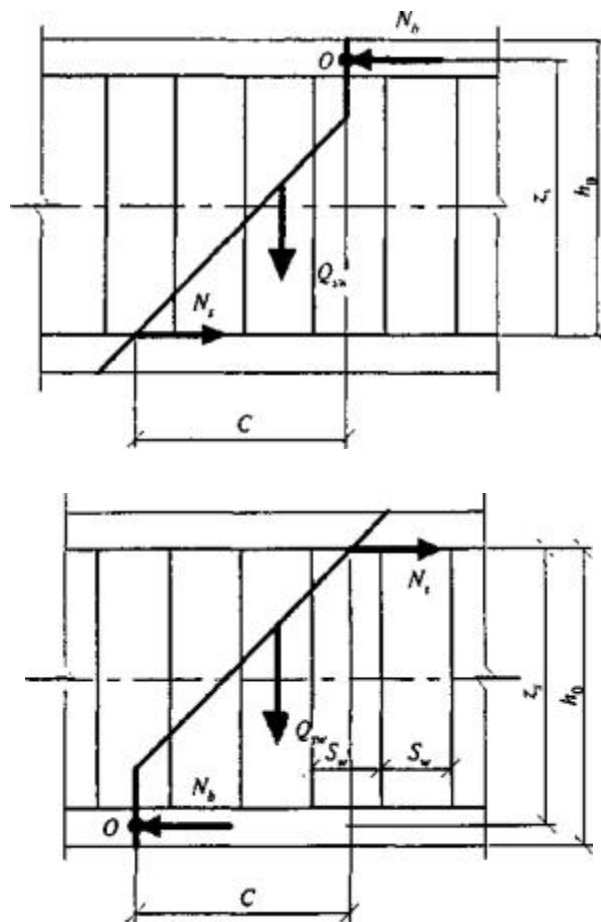
Рисунок 6.9 - Схема усилий при расчете железобетонных элементов по наклонному сечению на действие моментов
