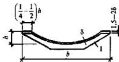
1 - ребра по поперечным краям элементов
