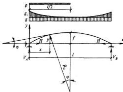
Рисунок 7.4 - Расчетная схема свода
