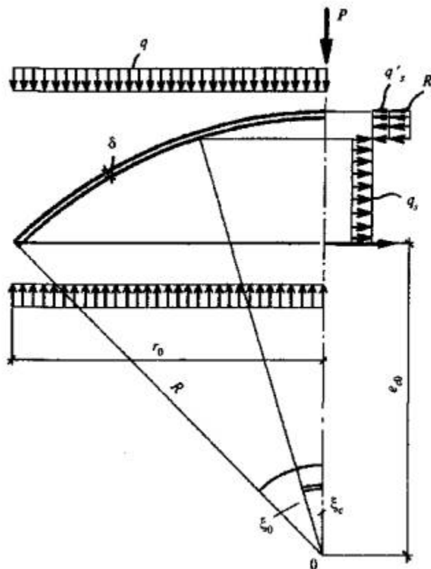
Рисунок 10.8 - К расчету купола по «балочной» схеме
