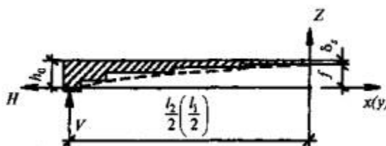
Рисунок 15.2 - Поперечное сечение и построение нижней поверхности ступенчато-вспарушенной панели
