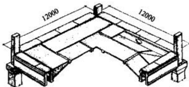
Рисунок 16.6 - Ячейка сборного шатрового перекрытия под тяжелые нагрузки
