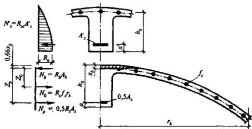
Рисунок 11.20 - Схема взаимодействия усилий в радиальном сечении оболочек
