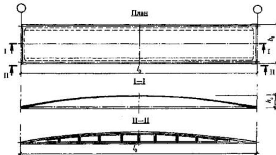
Рисунок 14.1 - Панель-оболочка КЖС
