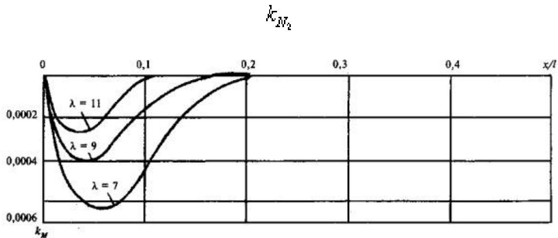
Рисунок 11.7 - Графики коэффициентов k_M
