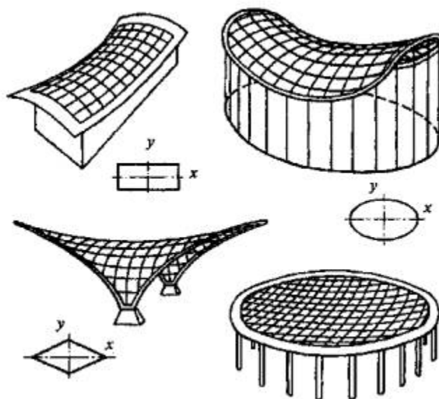
Рисунок 13.4 - Висячие оболочки с перекрестной системой вант
