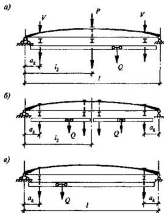
Рисунок 14.8 - Типовые схемы нагружения (а, б, в) покрытая из панелей-оболочек КЖС подвесными кранами
