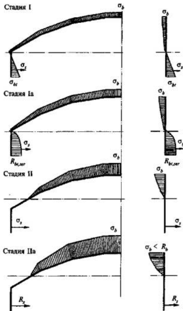
Рисунок 9.7 - Стадии напряженного состояния поперечных сечений оболочки (складки)
