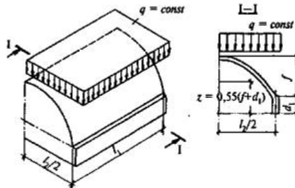
Рисунок 9.17 - К расчету бортового элемента короткой цилиндрической оболочки
