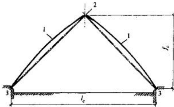
Рисунок 14.11 - Конструктивная схема сегментного свода для покрытий, опирающегося на продольные балки каркаса здания
