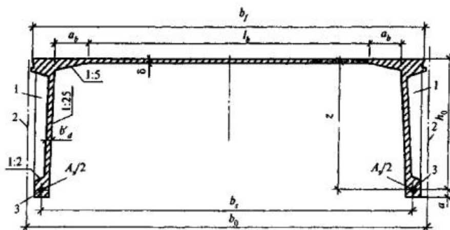
Рисунок 14.1 - Панель-оболочка КЖС
