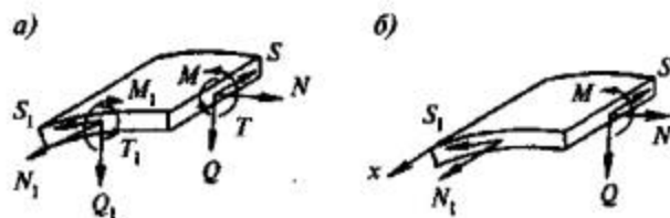
a - полная схема усилий; б - усилия, учитываемые при расчете
