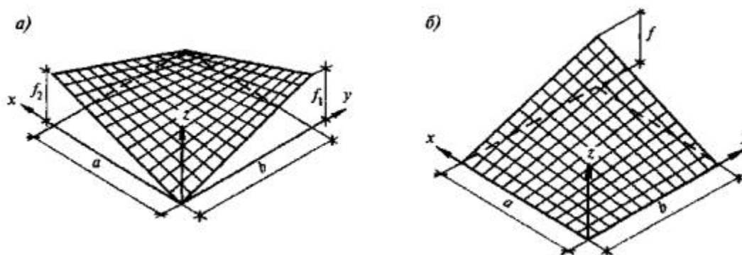
Рисунок 12.2 - Однолепестковые гипары
