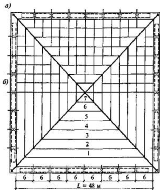
а - схема вантовой сети; б - схема железобетонной оболочки
