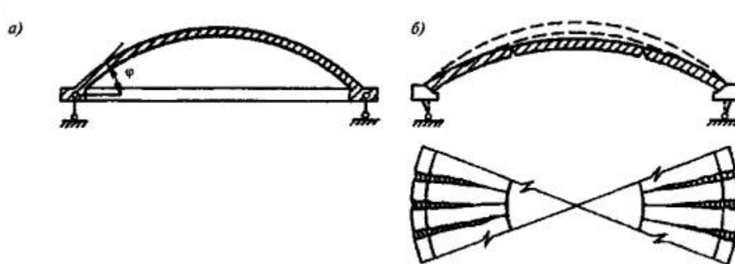
a - поперечное сечение; б - схема разрушения
