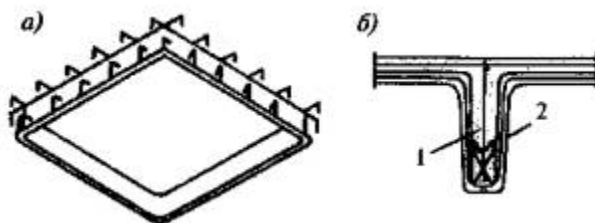
а - тонкостенный коробчатый железобетонный или армоцементный элемент; б - деталь поперечного сечения конструкции; 1 - монолитный бетон; 2 - выпуски арматуры из несущей опалубки
