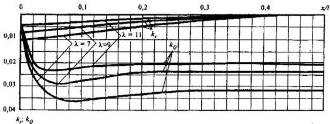
Рисунок 11.8 - Графики коэффициентов k_s, k_Q
