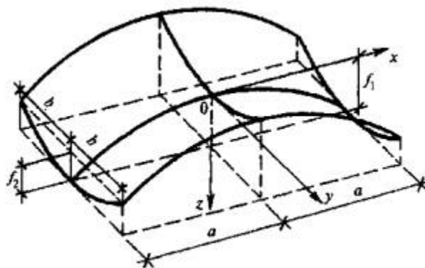
Рисунок 12.1 - Гиперболический параболоид
