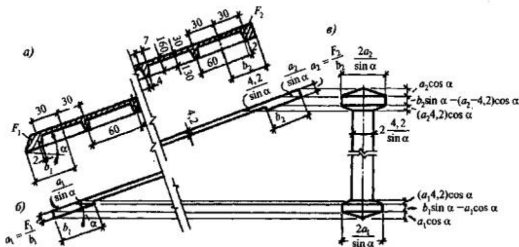
a - сечение панели свода; b - приведенное сечение панели; в - приведенное сечение складки свода
