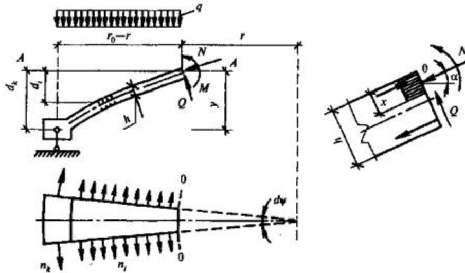
Рисунок 10.6 - Схема взаимодействия усилий в куполе в предельном состоянии
