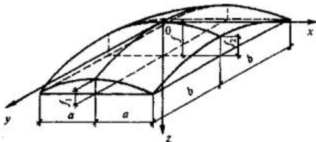
Рисунок 11.2 - Схема оболочки положительной гауссовой кривизны
