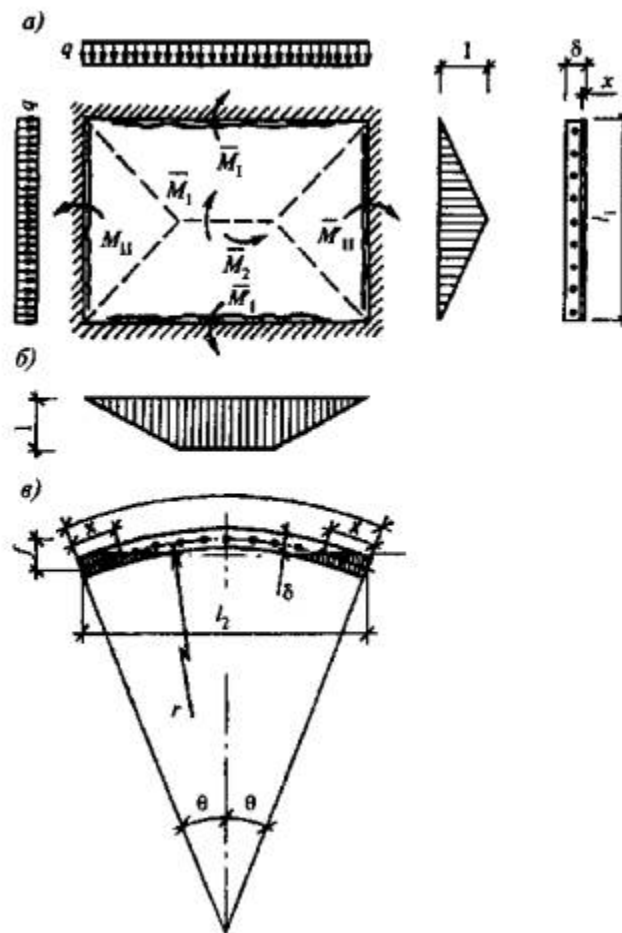
a - схема излома; б - перемещения панели в предельной стадии; в - сечение по криволинейному контуру панели
