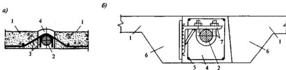
а - плоская плита; б - ребристая плита; 1 - железобетонная плита; 2 - ванта; 3 - крюки; 4 - бетон шва; 5 - армирование шва; 6 - ребро плиты; 7 - детали крепления плит к вантам
