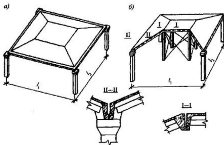
а - из шатровых элементов размером на ячейку здания; б - из унифицированных элементов с использованием сборочного кондуктора
