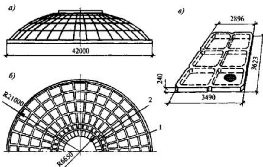
а - общий вид; б - план; в - трапециевидная плоская плита; 1 - монолитное нижнее опорное кольцо; 2 - монолитное верхнее опорное кольцо
