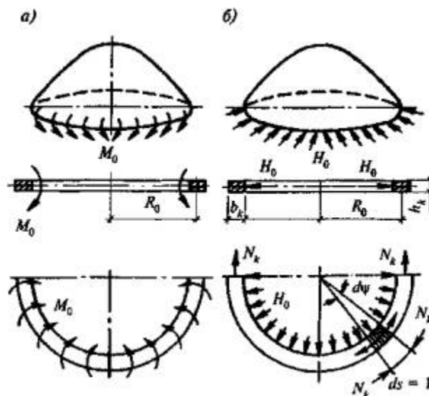
a - момент; б - распор
