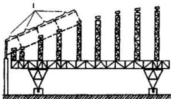
1 - укрупненные монтажные блоки
