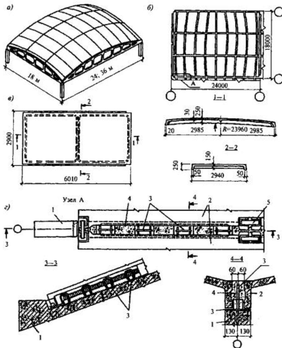
Рисунок 11.3 - Общий вид многоволновых сборных железобетонных оболочек положительной гауссовой кривизны
