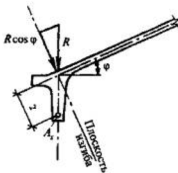
Рисунок 16.5 - Расчетная плоскость изгиба крайних элементов шатровых складок
