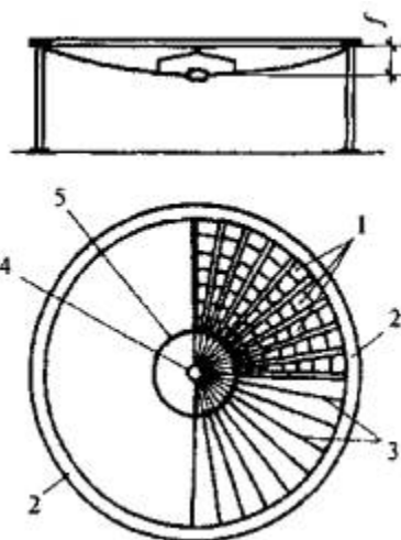
Рисунок 13.1 - Висячая оболочка с параллельной системой вант
