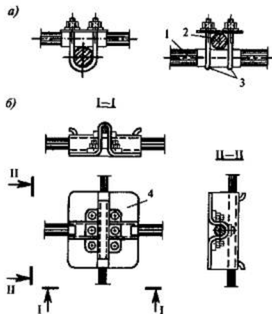
а - с применением хомутов; б - то же, штампованных стальных косынок; 1 - несущая ванта; 2 - натягающая ванта; 3 - хомут; 4 - косынка
