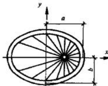
Рисунок 13.12 - Радиально-вантовая система с узлом в фокусе эллипса
