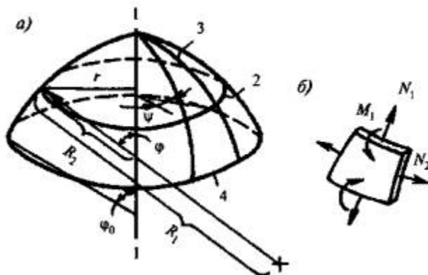
а - геометрия; б - схема усилий; 1 - ось вращения; 2 - параллель; 3 - меридиан; 4 - краевой параллельный круг
