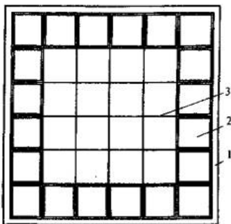
1 - опорный контур; 2 - плита; 3 - ванты
