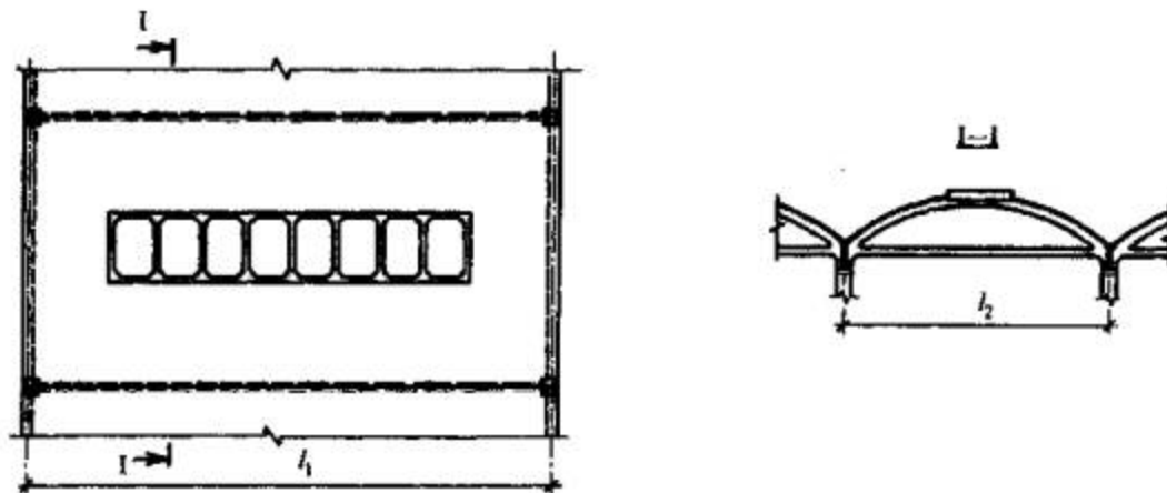
Рисунок 9.13 - Схема оболочки с фонарным проемом
