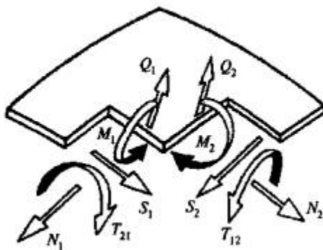
Рисунок 11.5 - Схема усилий в пологих оболочках
