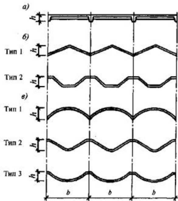
a - цилиндрические своды; б - складчатые своды (типы 1 и 2); в - волнистые своды (типы 1, 2, 3)
