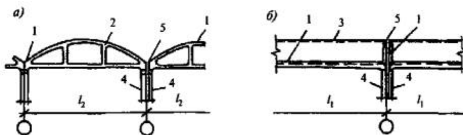
a - в направлении l_2 ; б - в направлении l_1 , 1 - бортовая балка; 2 - ферма-диафрагма; 3 - оболочка; 4 - колонна; 5 - шов
