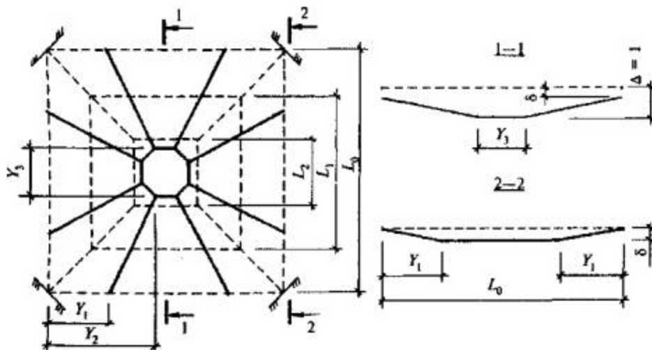
Рисунок 16.4 - Девятизвенная схема излома
