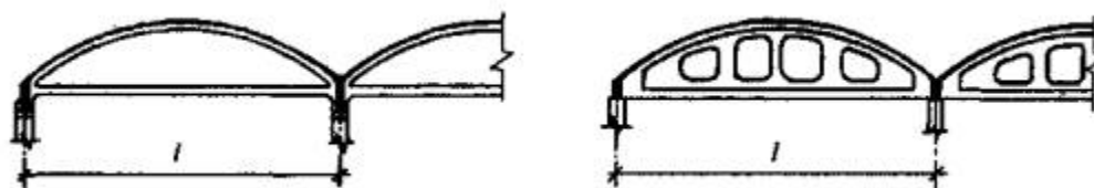
Рисунок 9.12 - Диафрагмы цилиндрических оболочек
