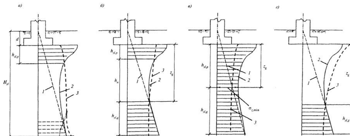
a - просадка от собственного веса s_{sl,g} отсутствует (не превышает 5 см), возможна только просадка от внешней нагрузки s_{sl,p} в верхней зоне просадки h_{sl,p} (I тип грунтовых условий); б , в , г - возможна просадка от собственного веса s_{sl,g} в нижней зоне просадки h_{sl,g} , начиная с глубины z_g (II тип грунтовых условий); б - верхняя и нижняя зоны просадки не сливаются, имеется нейтральная зона h_n ; в - верхняя и нижняя зоны просадки сливаются; г - просадка от внешней нагрузки отсутствует; 1 - вертикальные напряжения от собственного веса грунта \sigma_{zg} ; 2 - суммарные вертикальные напряжения от внешней нагрузки и собственного веса грунта \sigma_z = \sigma_{zp} + \sigma_{zg} ; 3 - изменение с глубиной начального просадочного давления p_s ; H_{sl} - толщина слоя просадочных грунтов (просадочная толщина); d - глубина заложения фундамента
