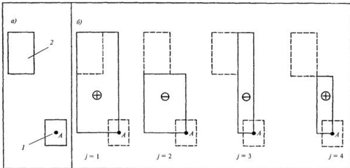
a - схема расположения рассчитываемого 1 и влияющего фундамента 2; б - схема расположения фиктивных фундаментов с указанием знака напряжений \sigma_{zp,cj} в формуле (5.19) под углом j -го фундамента
