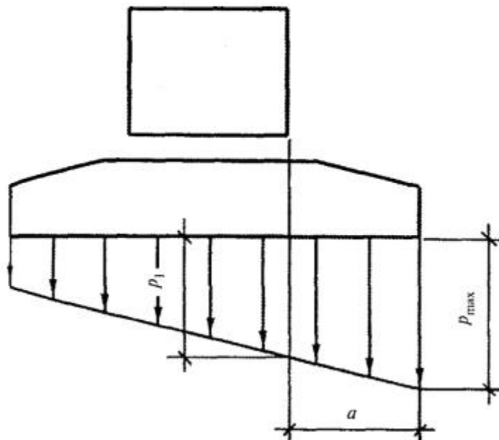
Рисунок 12.2. - К расчету ленточного фундамента
