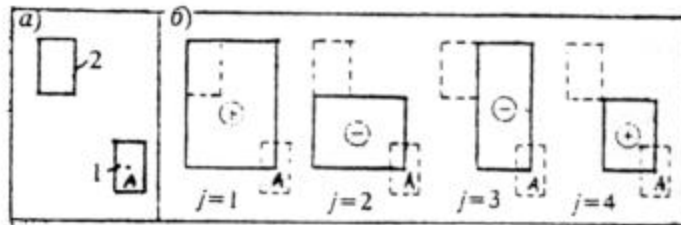
Рис. 2. Схема к определению дополнительных вертикальных напряжений s_{zp,a} в основании рассчитываемого фундамента с учетом влияния соседнего фундамента методом угловых точек
