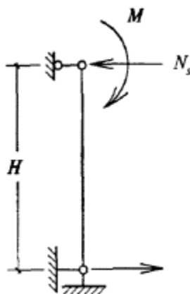
Рис. 12. Определение усилия в анкере от изгибающего момента в уровне перекрытия
