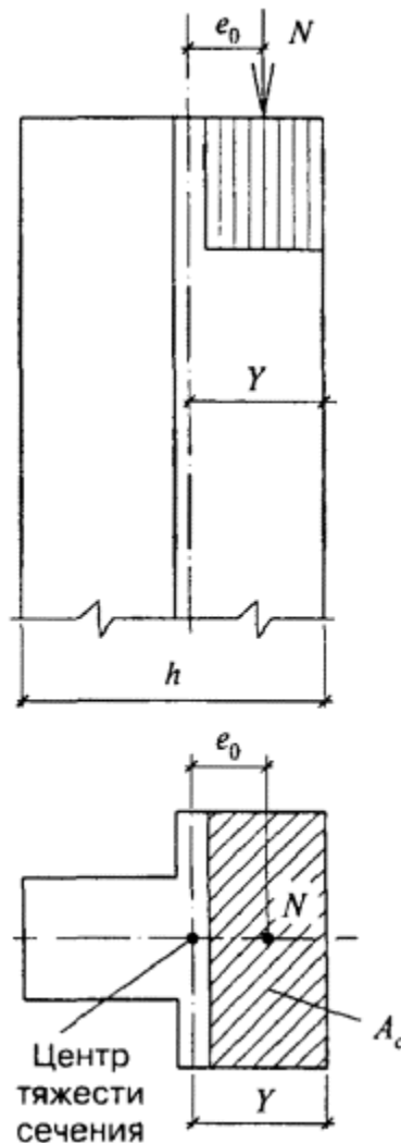
Рис. 5. Внецентренное сжатие
